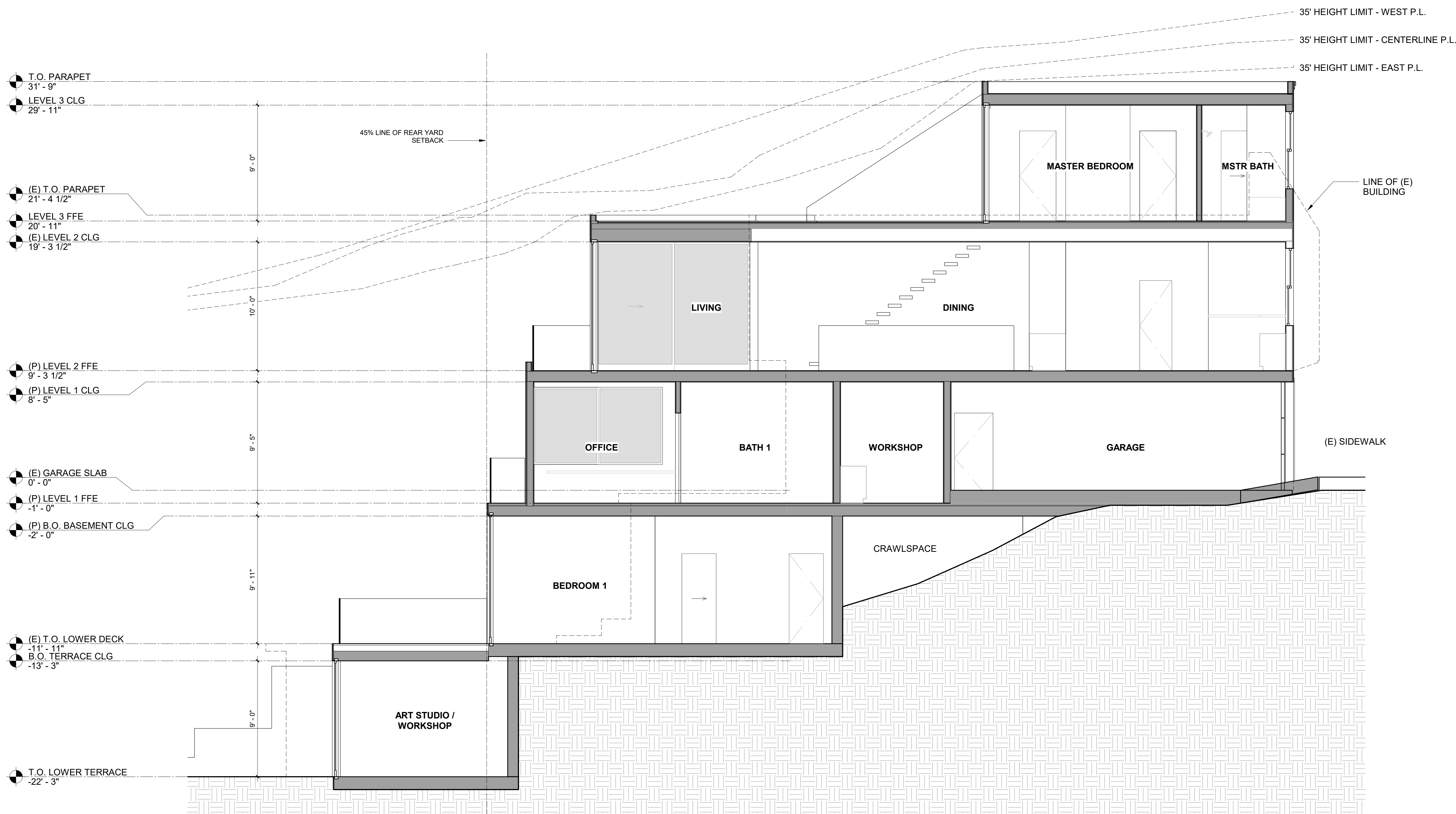
1 LONGITUDINAL SECTION 1 1/4" = 1'-0"
